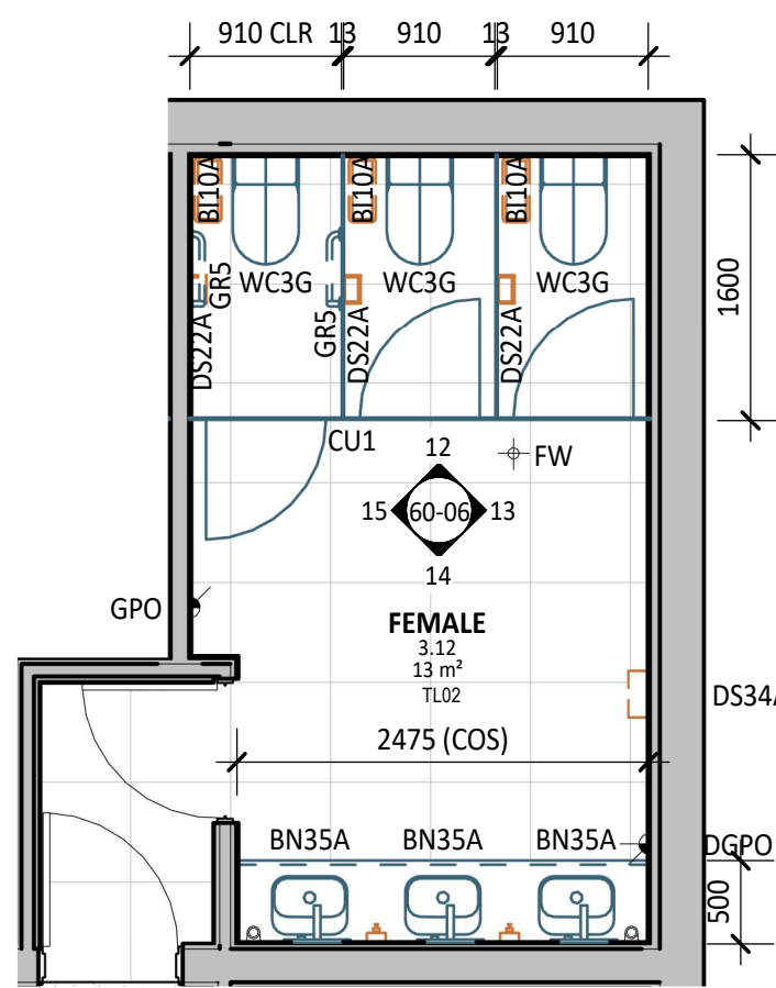
11 PLAN DETAIL 1 : 50
