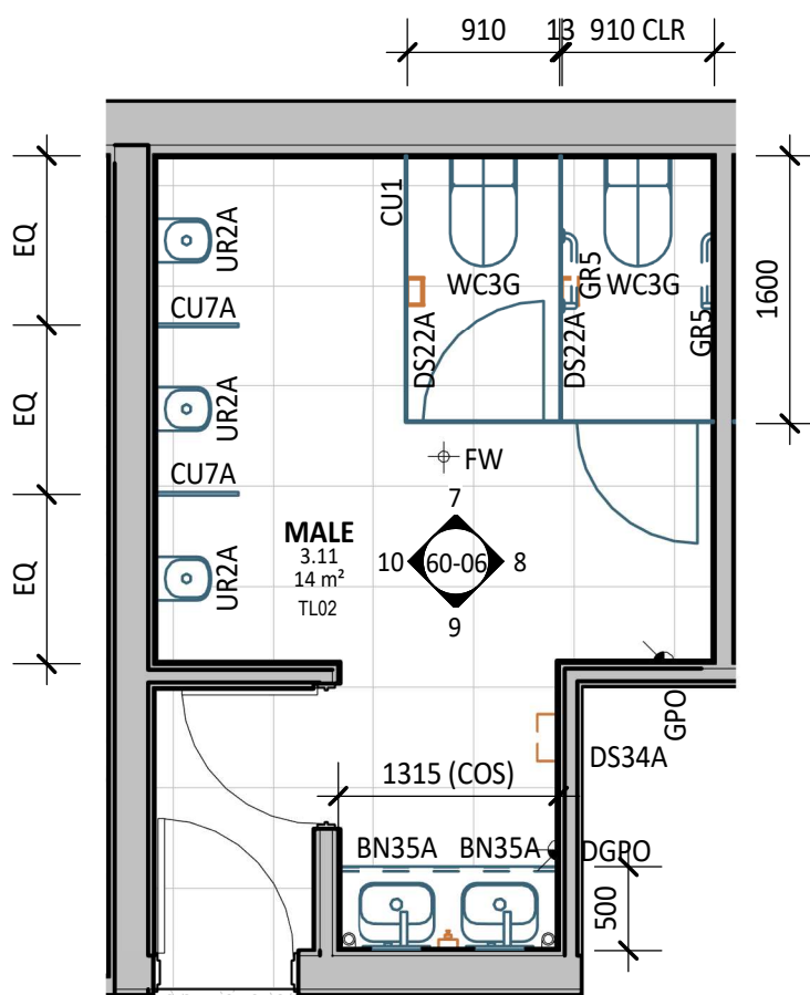
6 PLAN DETAIL 1 : 50
