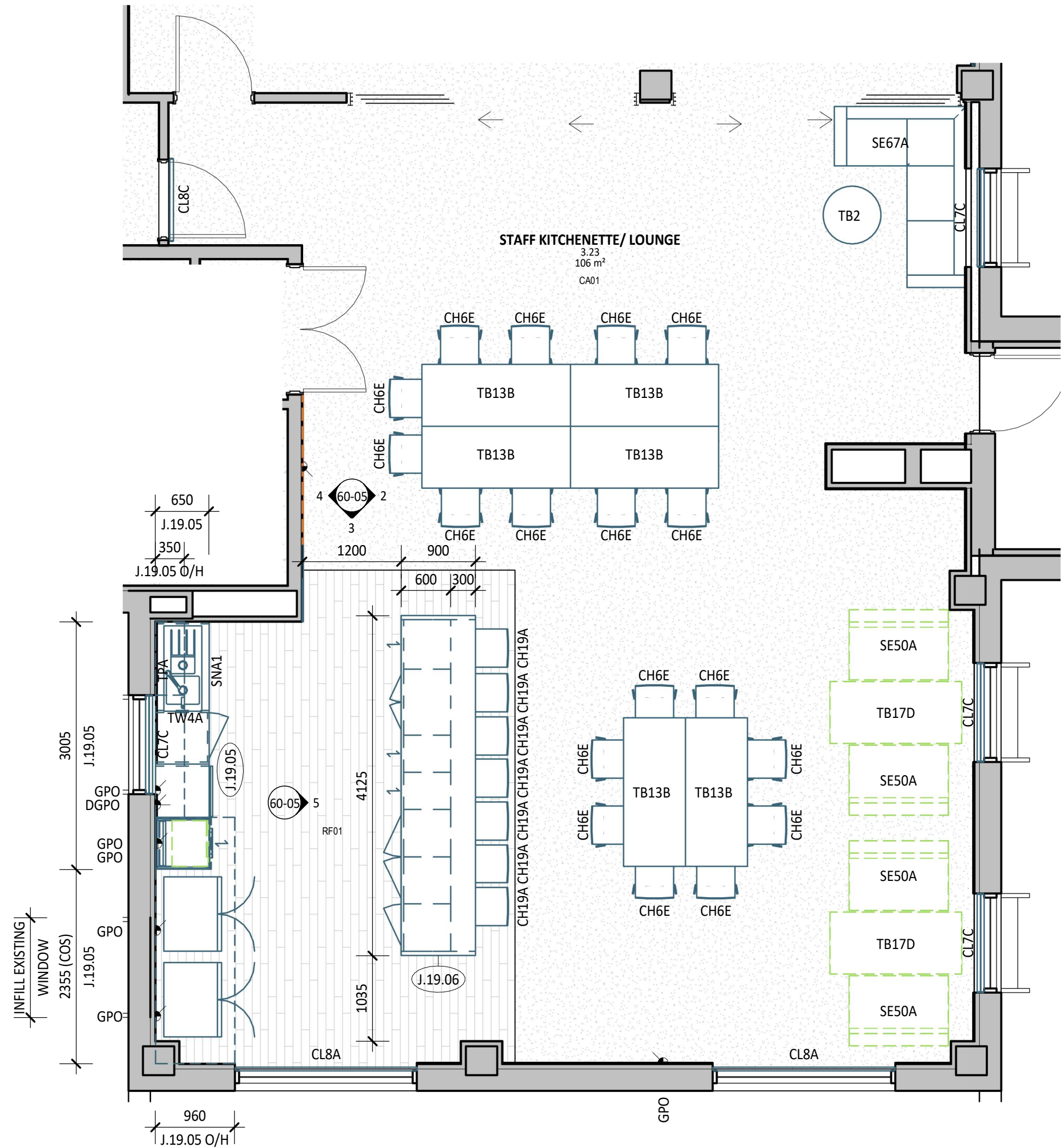
1 PLAN DETAIL 1 : 50
