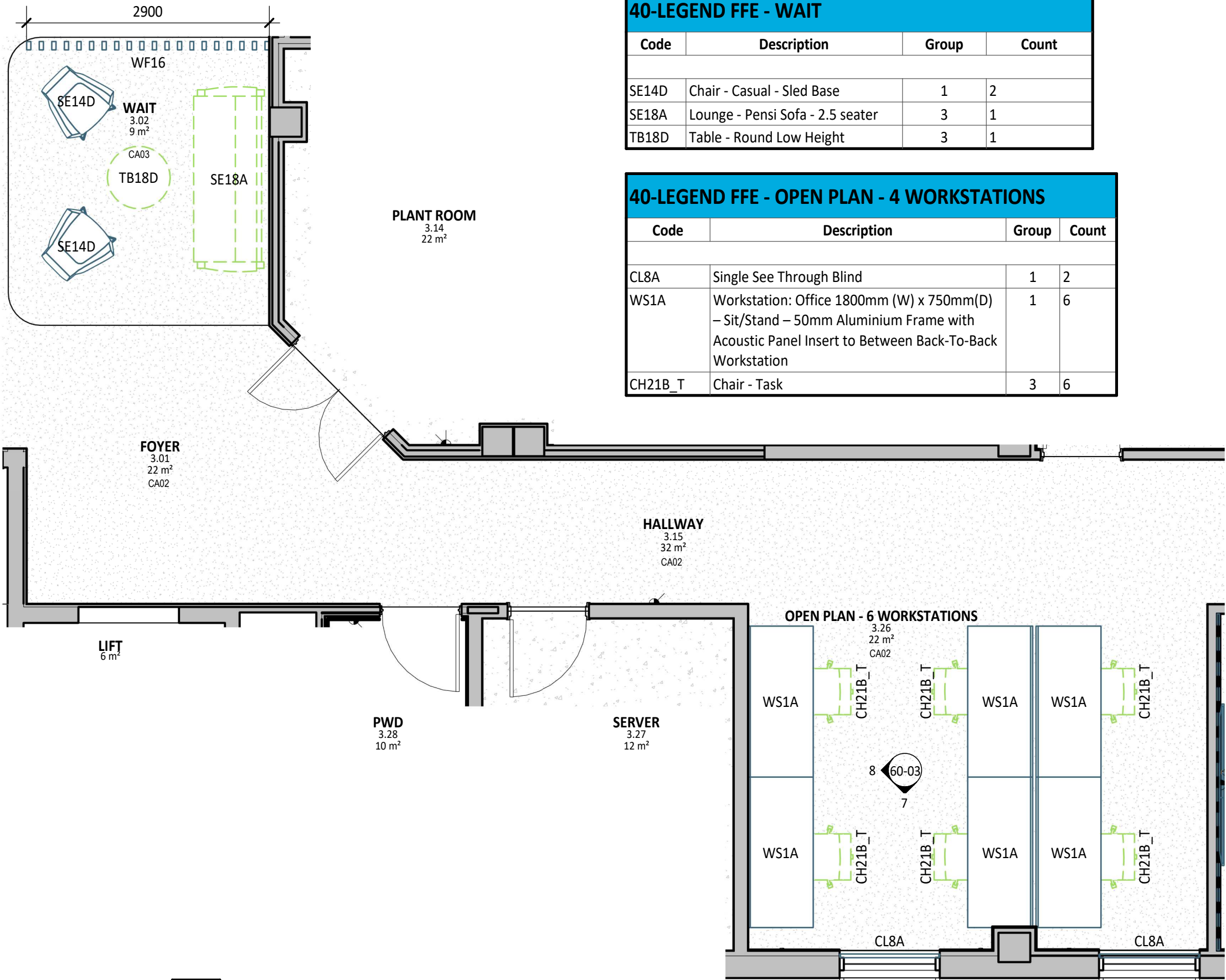
1 PLAN DETAIL 1 : 50
